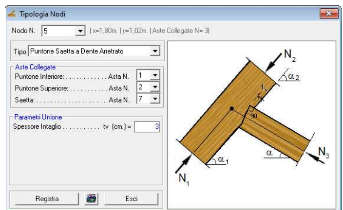
Puntone Saetta a Dente Arretrato
