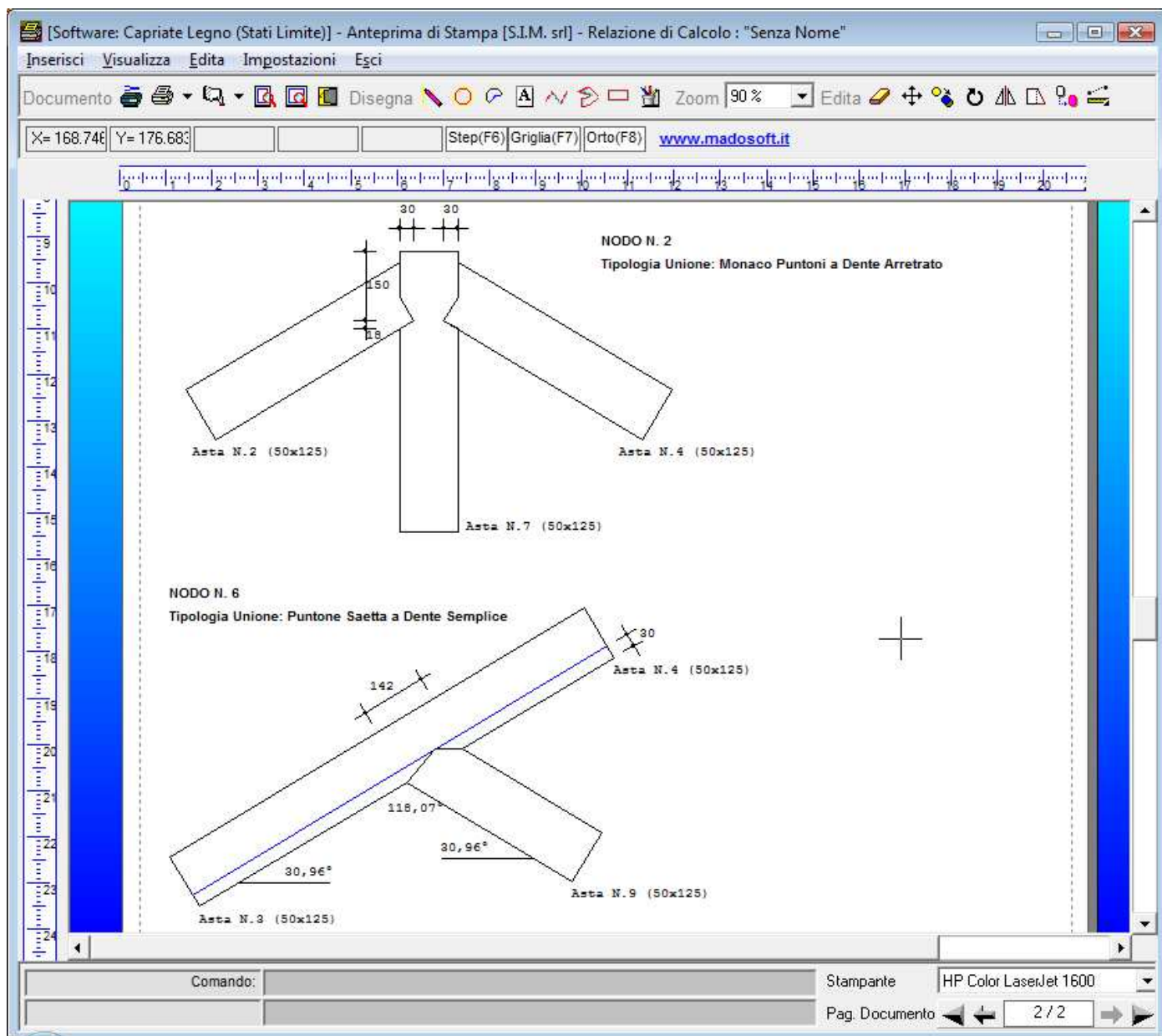
Figura 19 – Particolari costruttivi Collegamenti Aste
