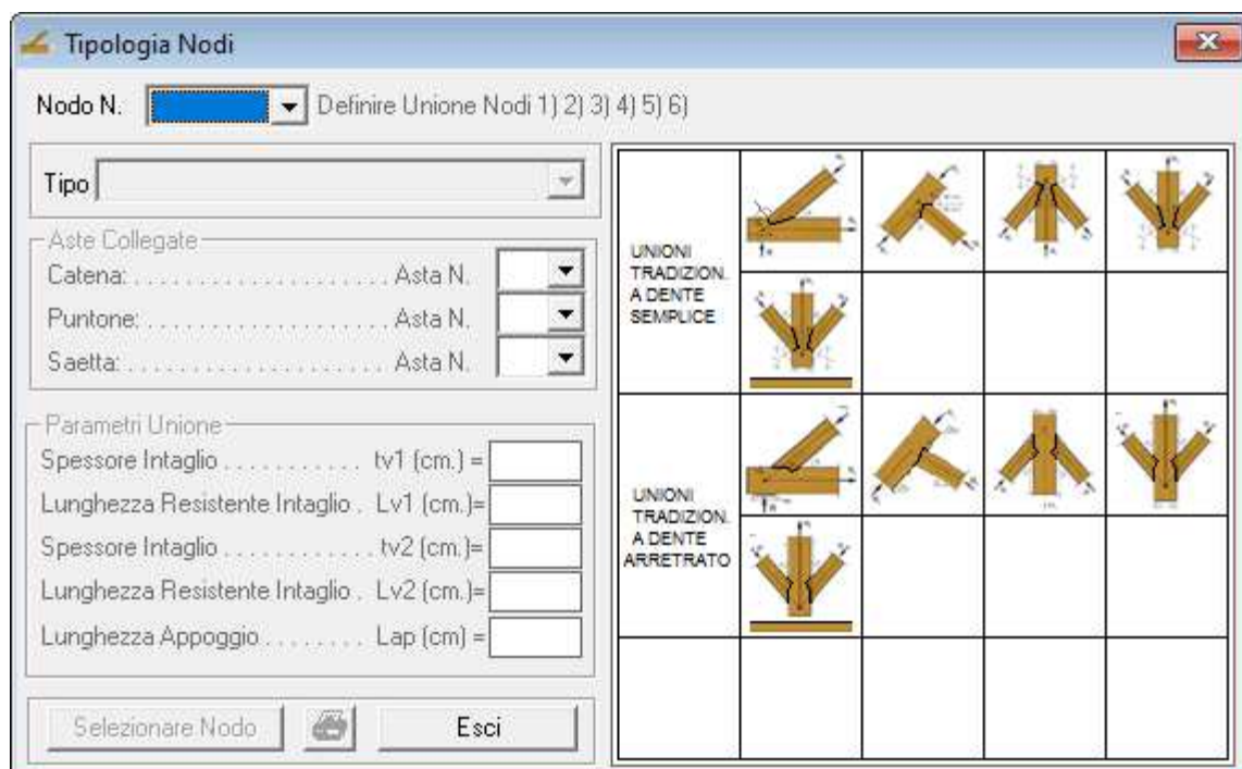
Figura 11 – Tipologia Nodi
