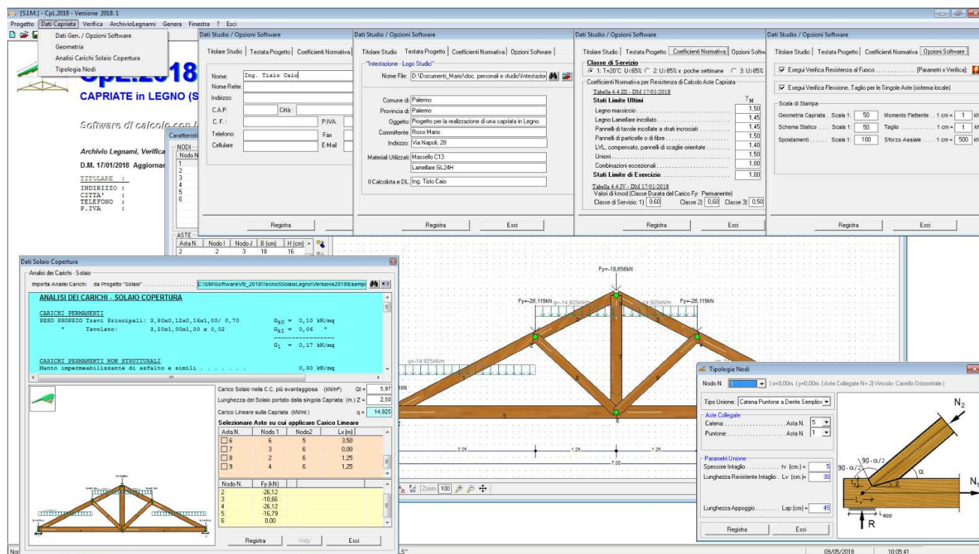
Figura 3 – Dati Capriata
