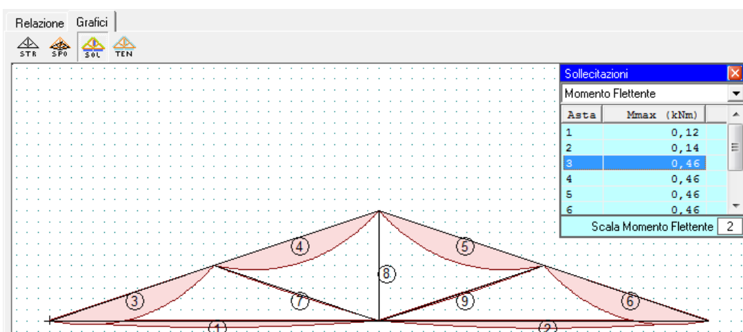
Figura 16 – Momento Flettente
