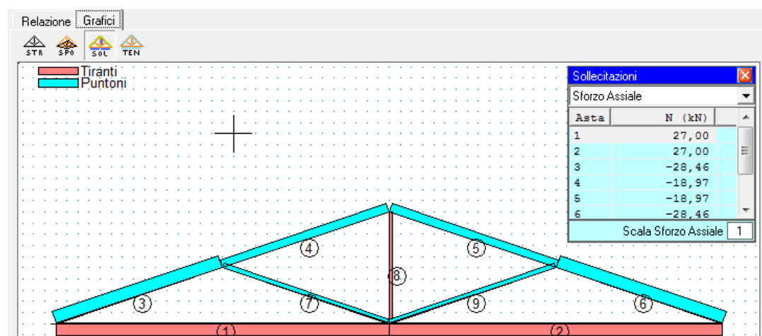
Figura 15 – Sforzo Assiale
