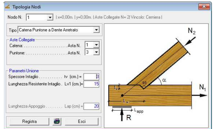
Catena Puntone a Dente Arretrato
