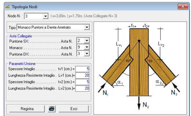
Monaco Puntoni a Dente Arretrato
