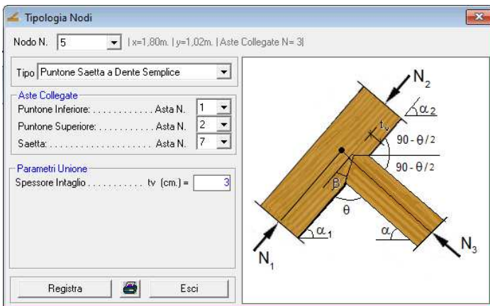
Puntone Saetta a Dente Semplice
