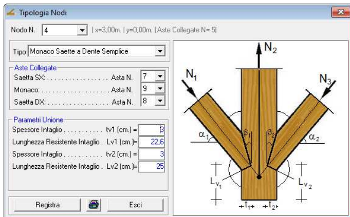
Monaco Saette a Dente Semplice
