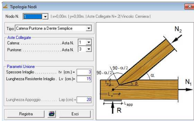
Catena Puntone a Dente Semplice
