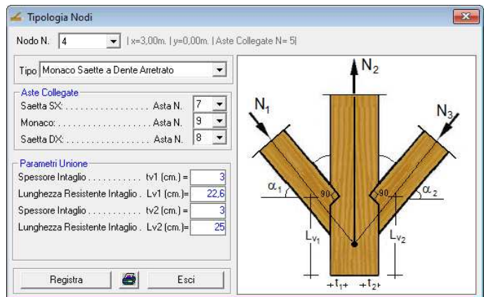
Monaco Saette a Dente Arretrato
