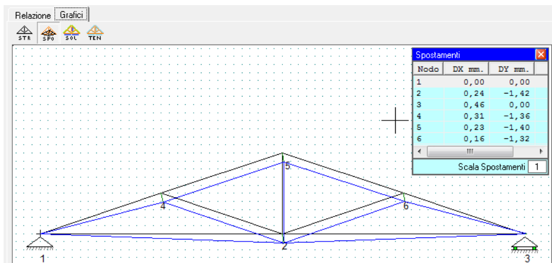
Figura 14 – Spostamenti
