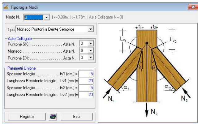
Monaco Puntoni a Dente Semplice
