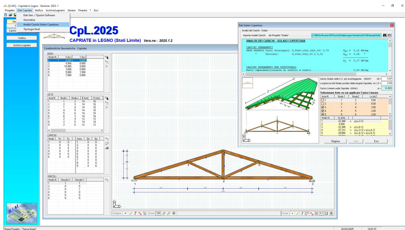
Figura 10 – Analisi dei Carichi
