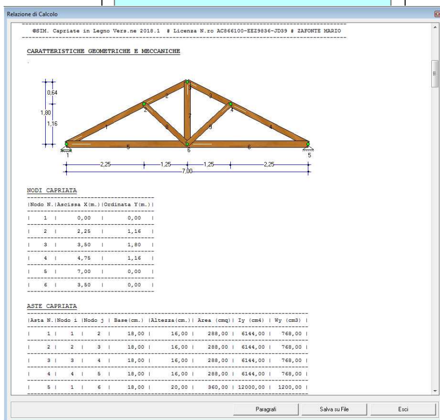
Figura 17 – Relazione di Calcolo
